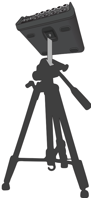
Abbildung 8. T4S mit Halterung auf dem Stativ anbringen
