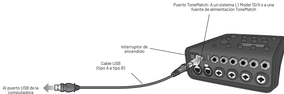
Figura 12. Conexión de T4S a USB
