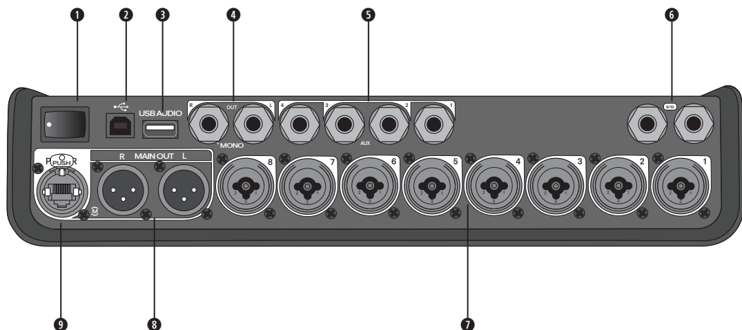
Figuur 4. T8S aansluitpaneel
