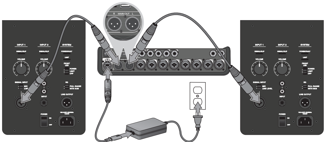
Figura 10 Due sistemi F1 collegati a un mixer T8S tramite connessione analogica
