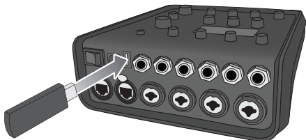
Figura 13. Conexión de una unidad flash al T4S
