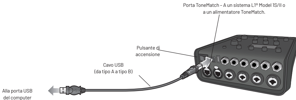
Figura 12 Connessione del mixer T4S alla porta USB
